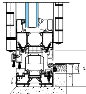
Ouverture extérieure : seuil PMR encastré
